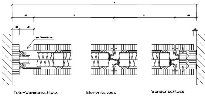
Tele-Wandanschluss
